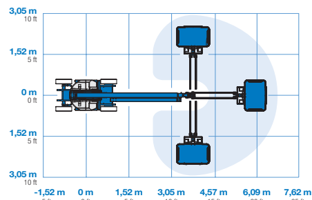
Courbe de travail Z-30/20N RJ
