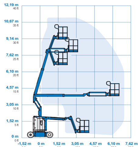
Courbe de travail Z-30/20N RJ
