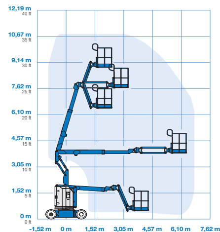
Courbe de travail Z-30/20N RJ
